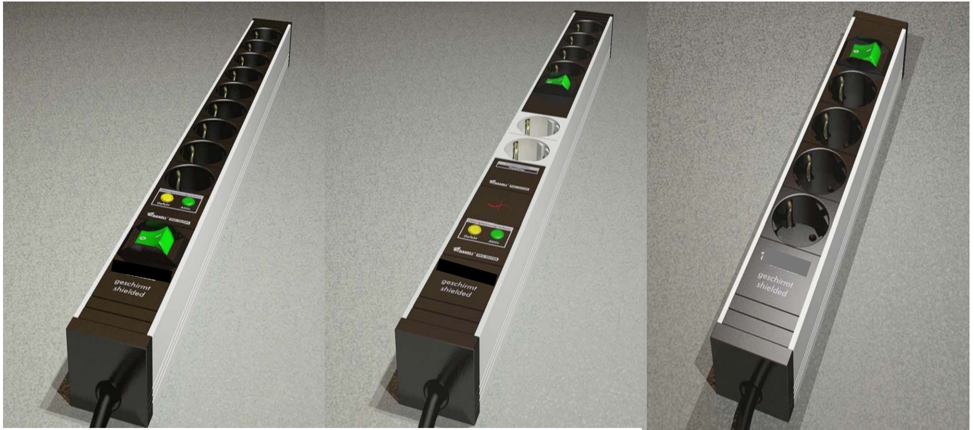
41-6788 Steckdosenleiste, 9-fach, Schalter 2-polig, ÜSS (Überspannungsschutz), Kinderschutz, 3m Kabel, VDE-Zeichen
